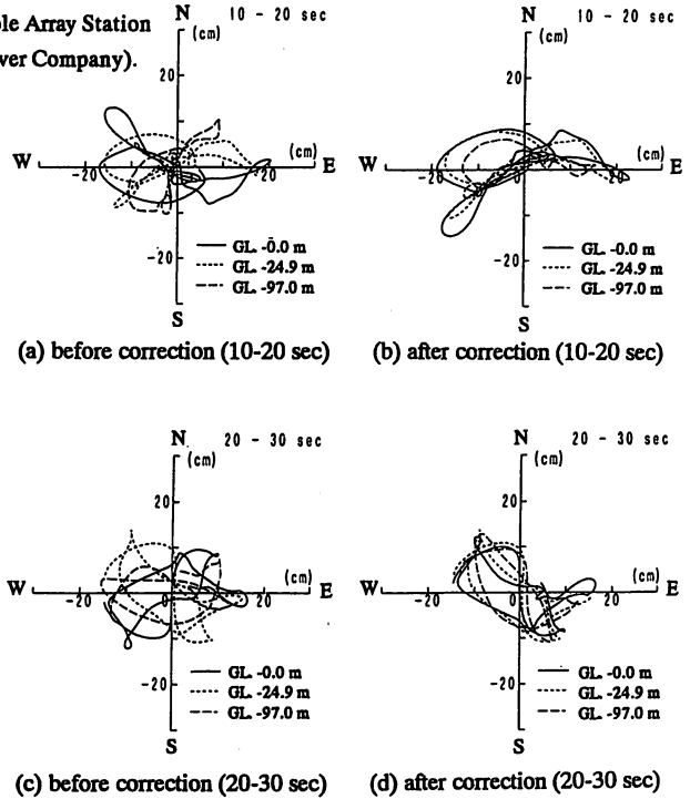
Fig. 5 Displacement Orbits
