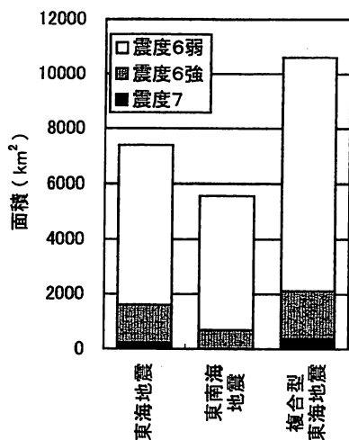
図12 震度階別面積の比較(東海4件)
