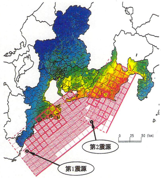
(c) 複合型東海地震
