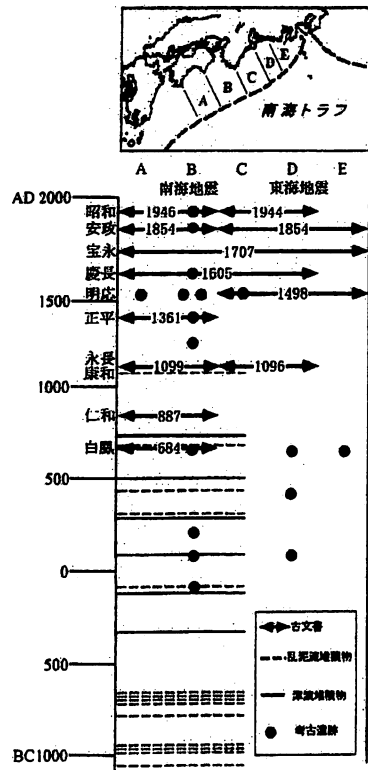
図1 南海トラフ域における過去3000年の巨大地震の発生状況 1)
