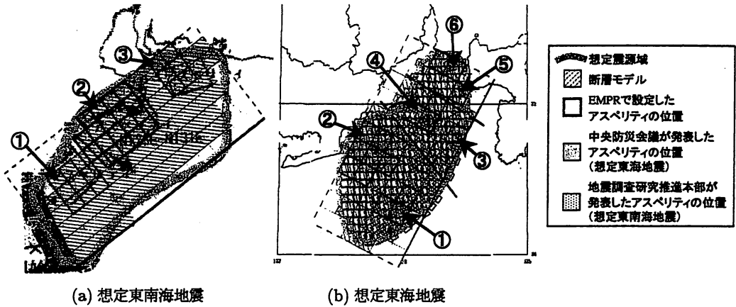
図4 東海地震の震源域とアスペリティの位置(文献 2),3 )に加筆
