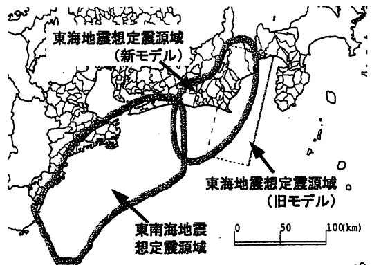
図2 東海地震、東南海地震の想定震源域
